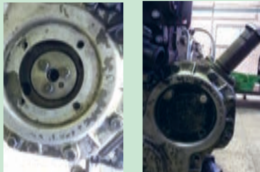
شکل ۳۲. پیچ های درپوش زمان بندی و چرخنده پمپ انژکتور تراکتور MF285
