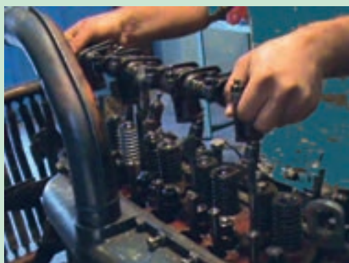
شکل ۴۶. برداشتن مجموعه اسبک از روی سرسیلندر
