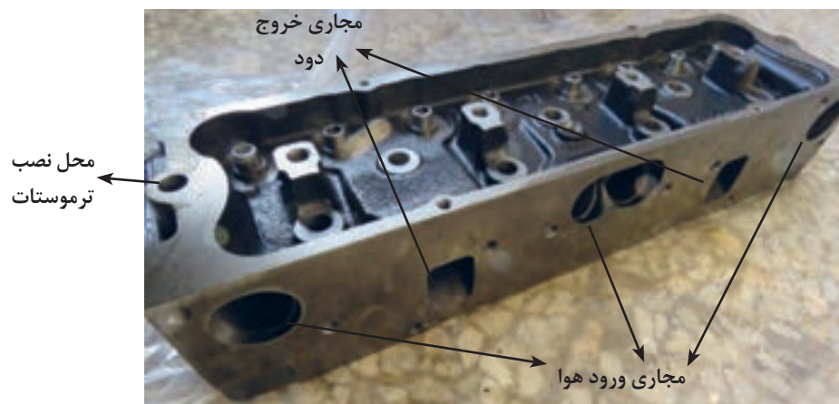
شکل ۱۱. سرسیلندر تراکتور MF۲۸۵ از دو نمای مختلف
