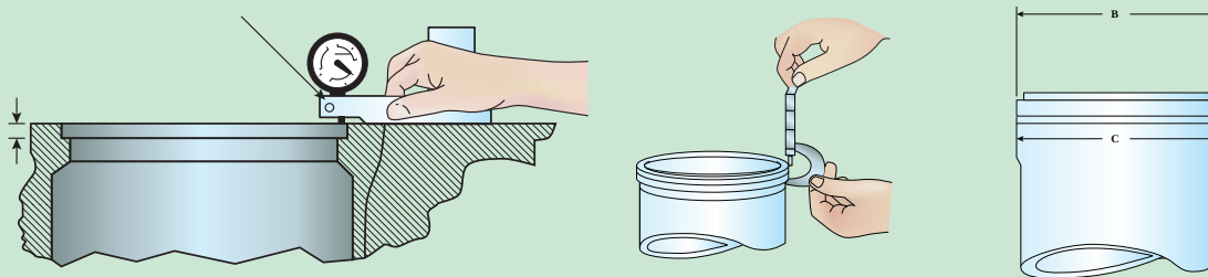
شکل ۸۹. اندازه گیری لبه بوش و جای آن در بلوکه سیلندر
