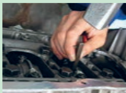
شکل ۴۱. علامت زدن کپه شاتون
