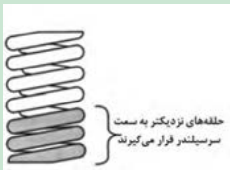
شکل ۸۵. جهت نصب فنر سوپاپ
