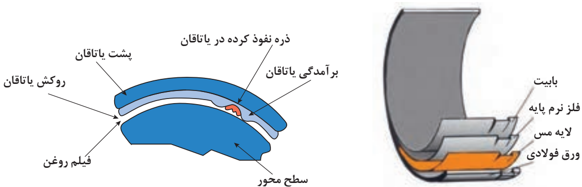
شکل ۱۹. انواع لایه بندی یاتاقان
