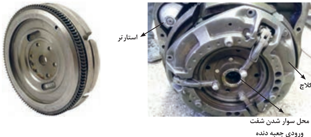
شکل ۲۶. فلایویل و قطعات متصل به آن
